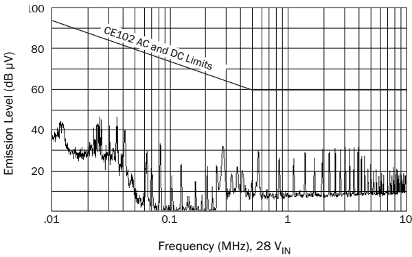
SMRT Dual MIL-STD-461 D-F, CE102
