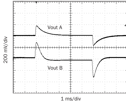
Load 50 - 100 - 50%, 50 Vin
