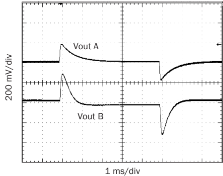
Load 50 - 100 - 50%, 28 Vin
