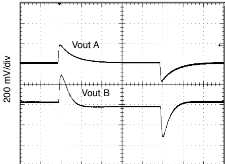
1 ms/div Load 50 - 100 - 50%, 28 Vin
