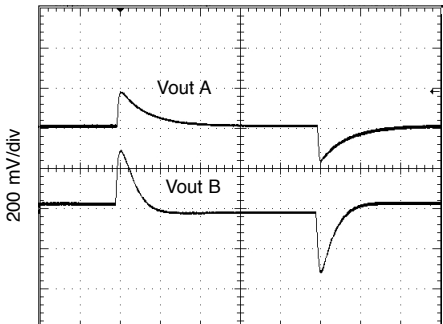
1 ms/div Load 50 - 100 - 50%, 50 Vin
